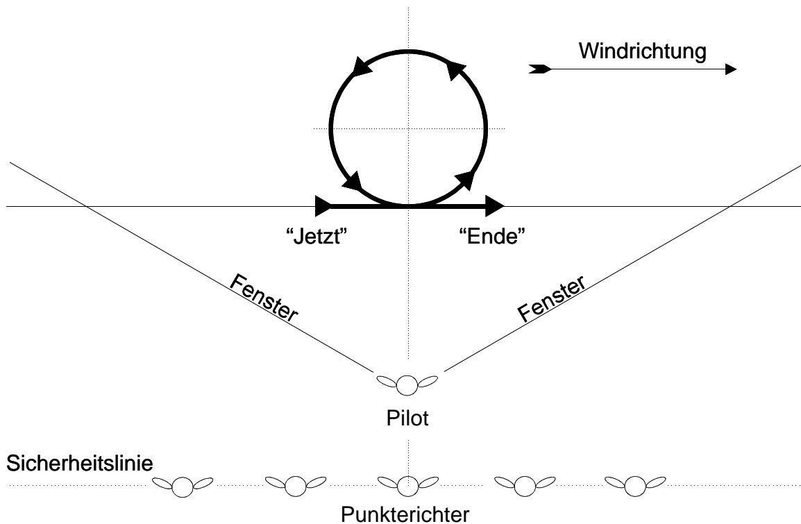
15.10.7.4 Figur 4 Verfahrenskurve
