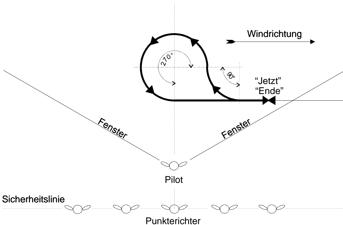
15.10.7.4 Figur 4 Verfahrenskurve
